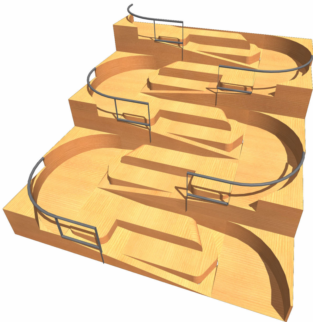
La rampa - escalera
